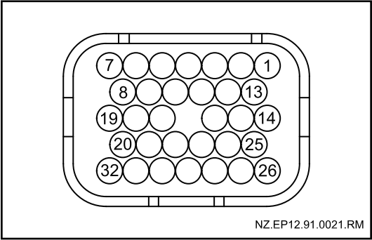
端子图
